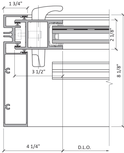
1 JAMB DETAIL
