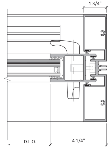
3 JAMB DETAIL
