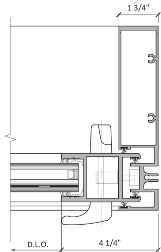
6 JAMB DETAIL
